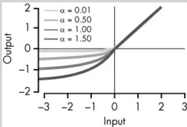
ELU
