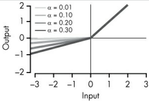
PReLU
